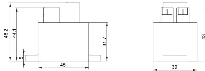
外形图
