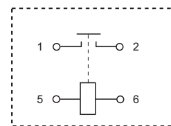
接线图
